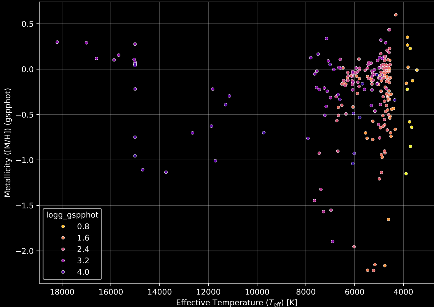
APOGEE DR17 Field: [131+00] Stellar Population Parameters (n= 250)
